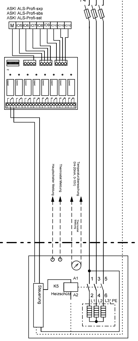
Geräte mit Optimierungskontakt (optional mit Rückmeldungen, Temp.überwachung)
