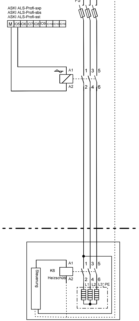
elektronischer Halbleiterschütz (2 oder 3 pol)
